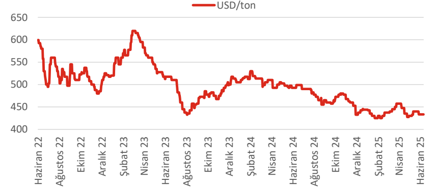
Kütük- FOB Rusya çıkışı
